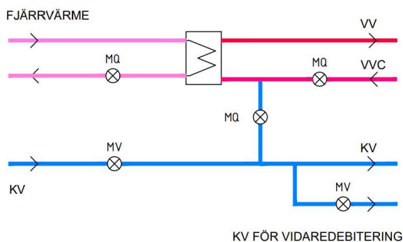
Figur 7. Exempel på volymmätning för tappvatten.
